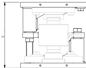
Capteur et plaques vendu séparément Load cell and plates sold separately
